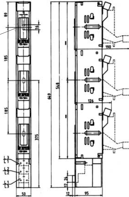
NH-Sicherungs-Lastschaltleiste Gr. 00/185: 125/160 A NH fuse-switch, vertical design, size 00/185: 125/160 A
