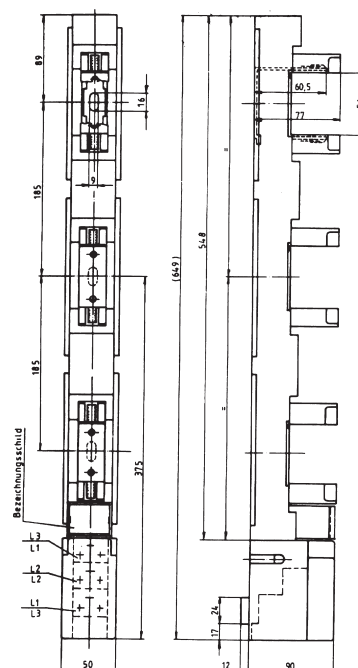
mit Kontakt- und Anschlußraumabdeckung with contact- and terminal-cover
